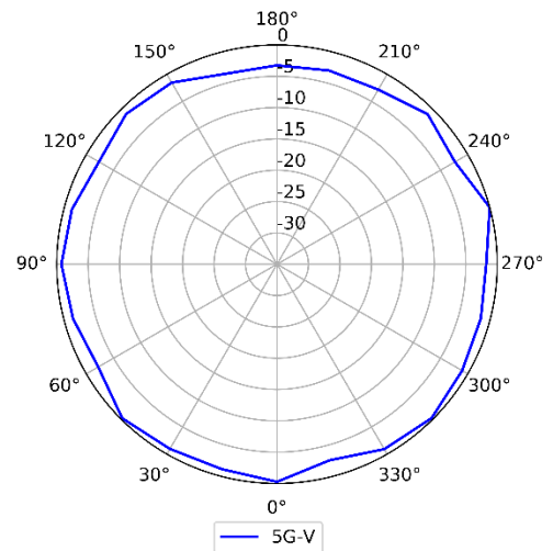
5GHz (Vertical)
