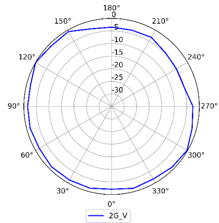
2.4GHz (Vertical)
