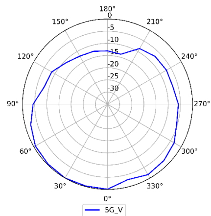
5GHz (Vertical)
